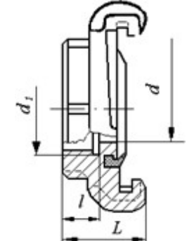
Рис. 4. Конструкция головки соединительной напорной ГМ-50П
